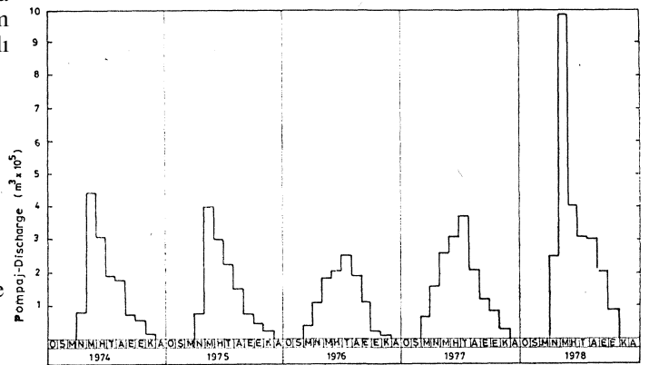
Şekil 6. Dört Yol kooperatif kuyularından toplam aylık pompaj dağılımı
