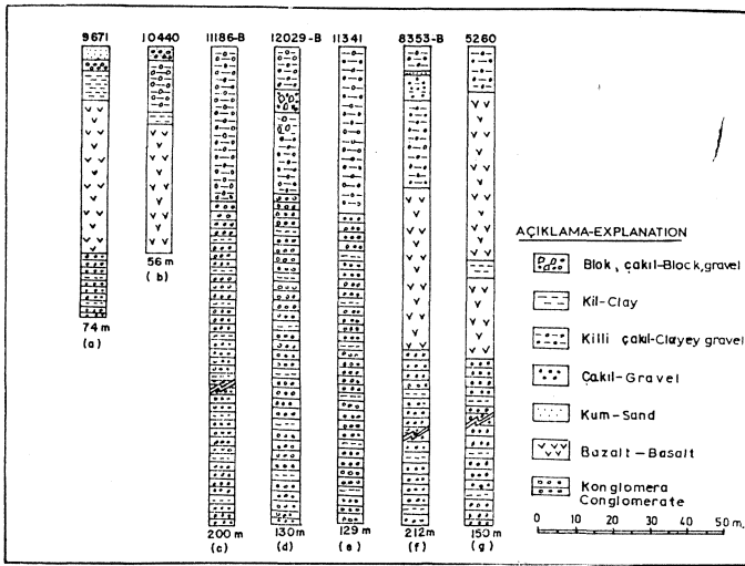
Şekil 7. Erzin ve Dört Yol ovalarından seçilmiş gözlem kuyularına ait loglar.
